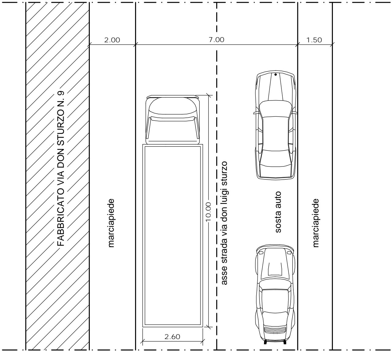
planimetria - scala 1:100 Monza via Don Luigi Sturzo n. 9
