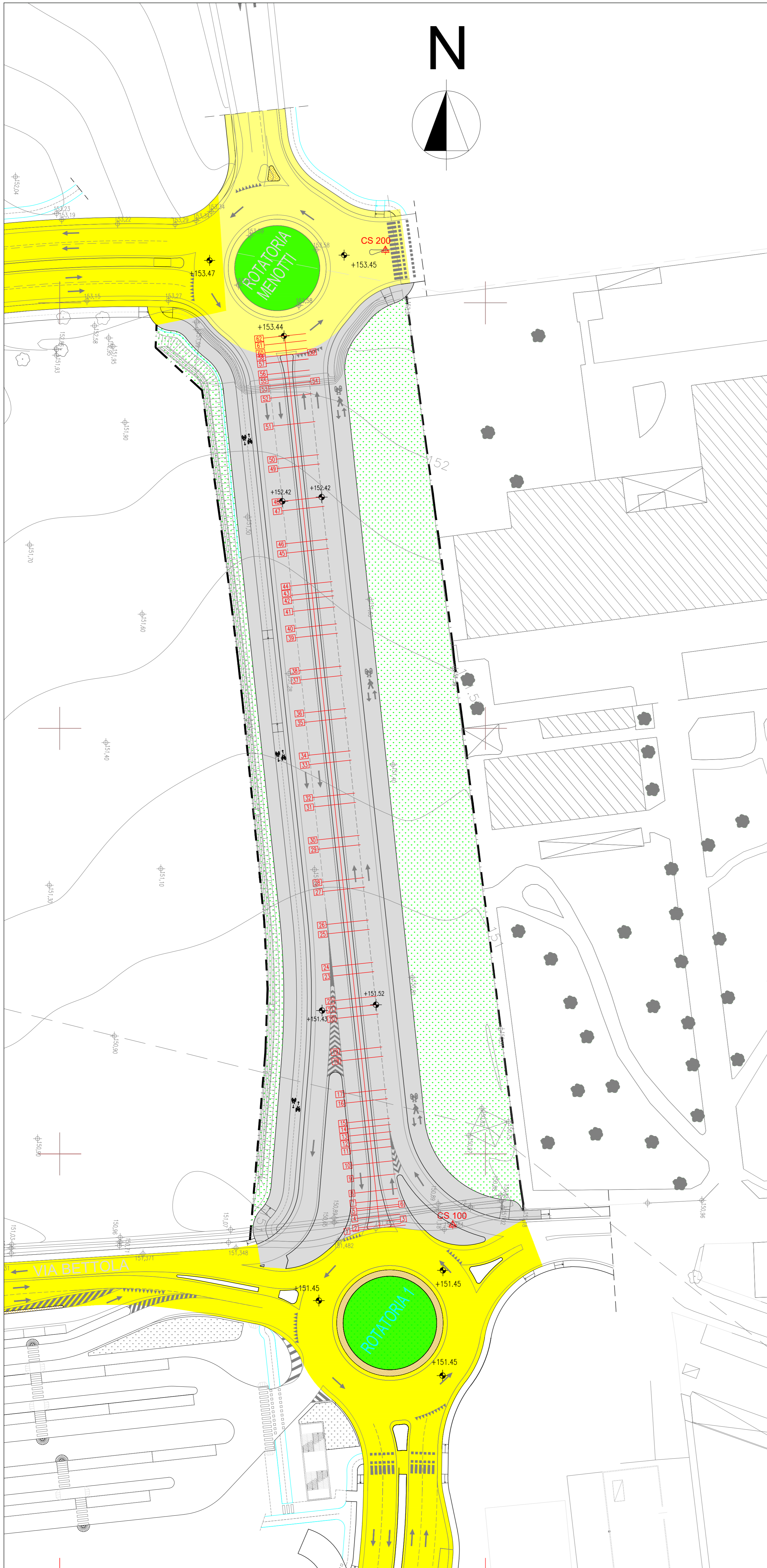
PLANIMETRIA TRONCO
