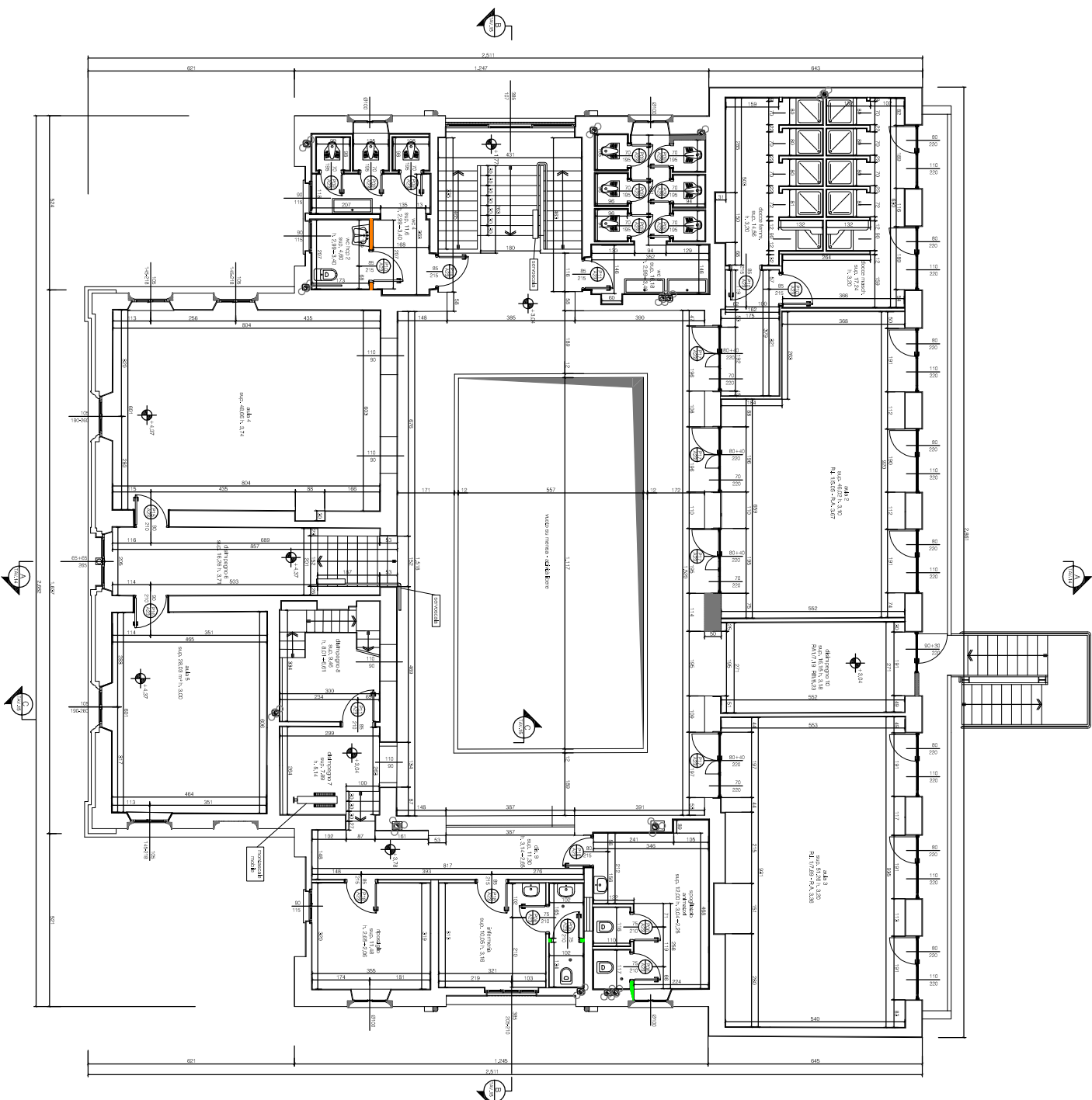
PIANO PRIMO
